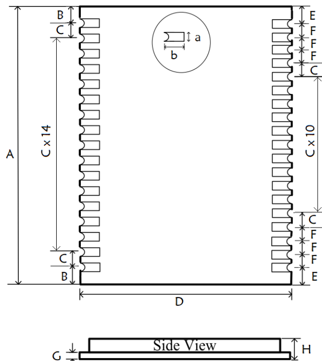
图 2 结构尺寸图
