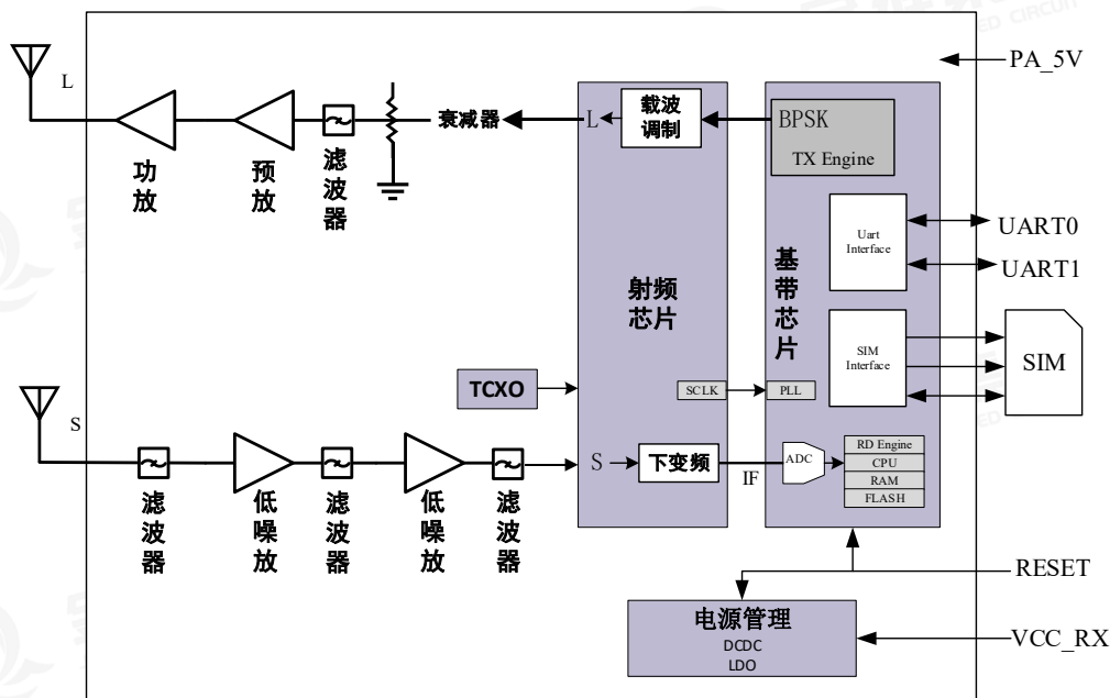
图 1 DM222 原理框图
