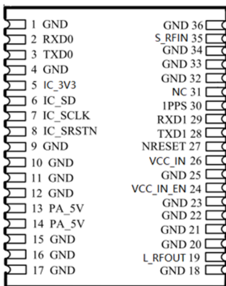
图 4 引脚定义图
