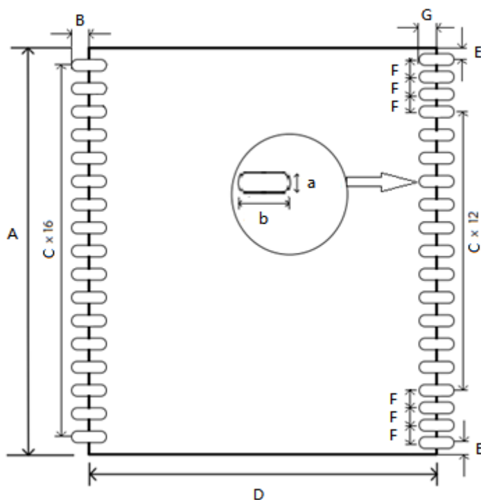
图 3 封装尺寸图
