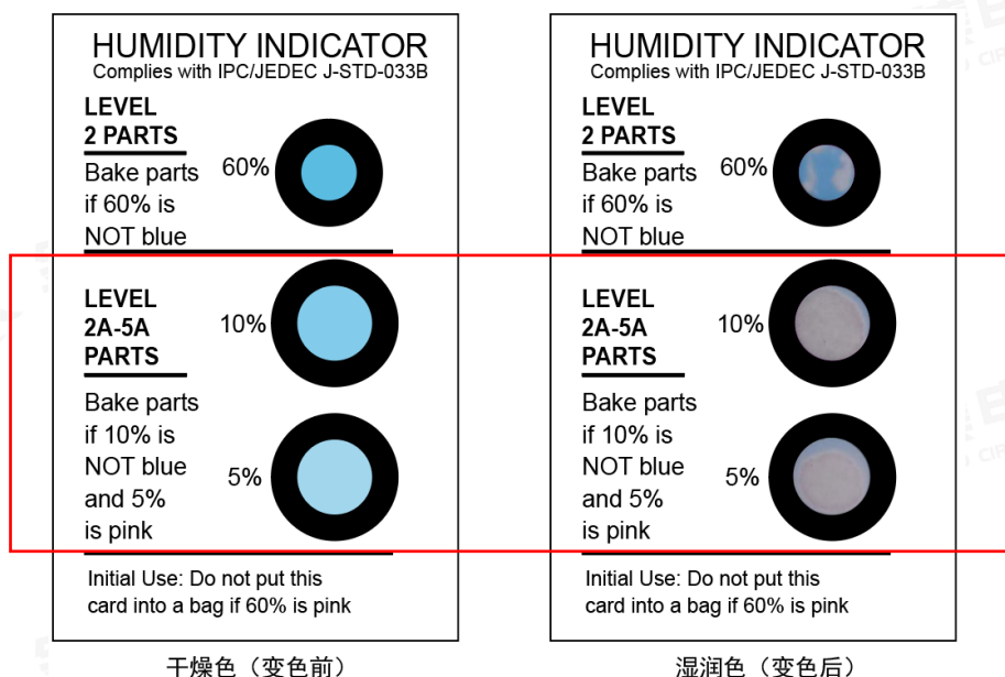
图 7 防潮标识卡 (三点湿度指示卡)
